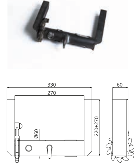
Verricello tendifune con tubino e asola Ø60 Winches with pipe and buttonhole Ø60
