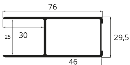
Montante VIP2 perno orizzontale senza battuta / Aluminium lock VIP2 with side pin, without wing
