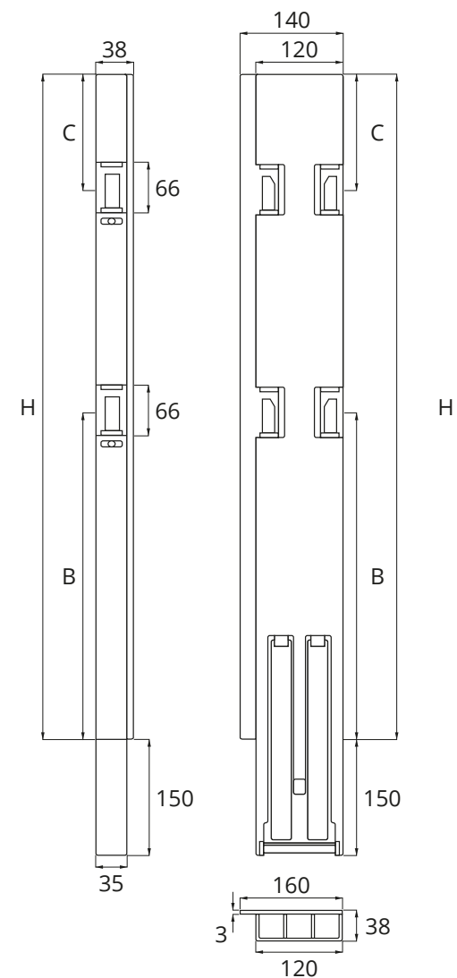
Montante posteriore sinistro Left rear pillar
