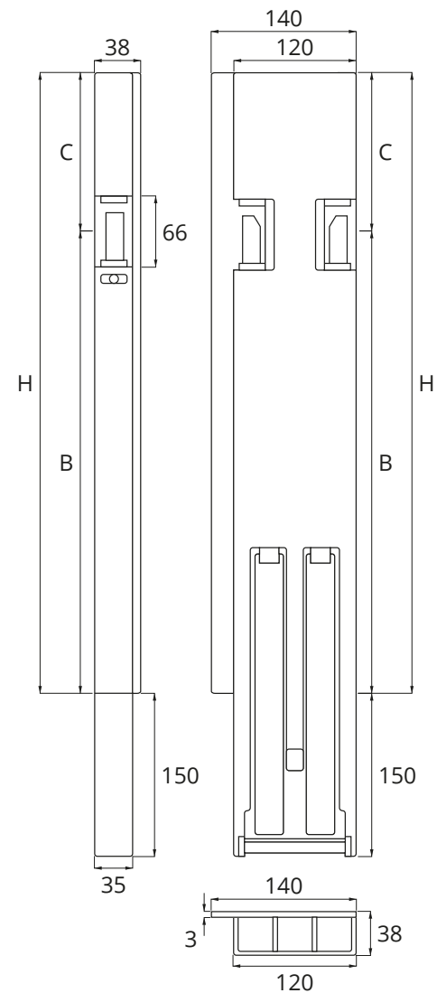
Montante posteriore sinistro Left rear pillar
